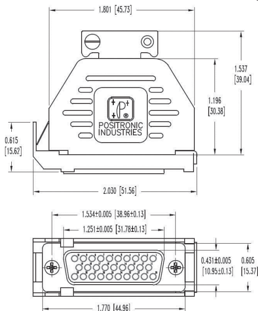
ALTO PN 200460 Positronic RD29S10JVLX Qty 1
